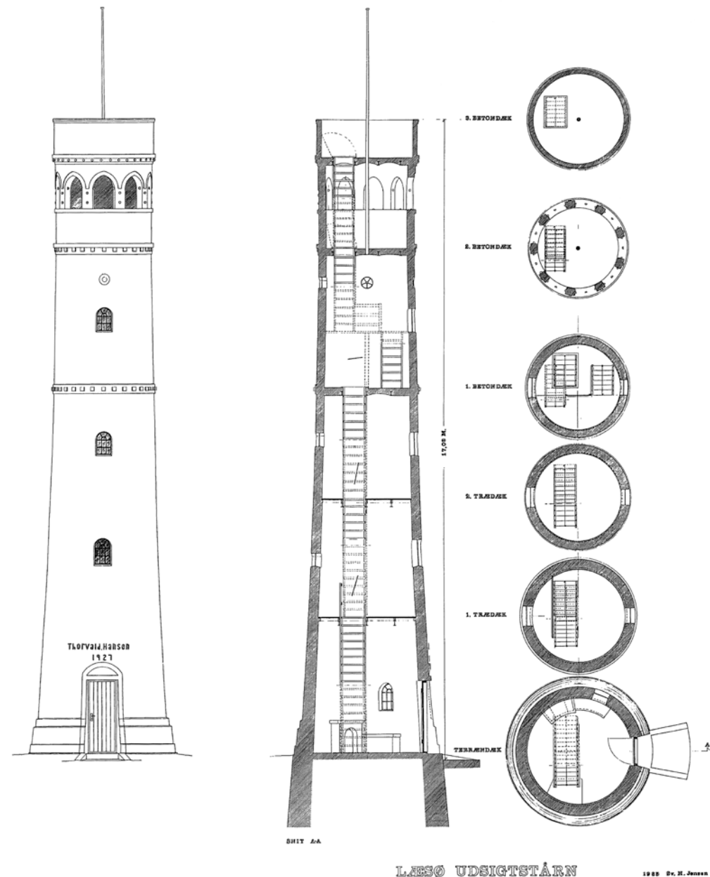
Detaliltegnning af tårnet fra 1985, der viser trapper og reposer, udsmykning og proportioner. Højde 17 meter. Signeret Sv. H. Jensen.
